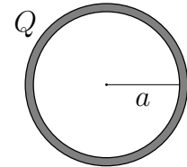
図1 一様に帯電した球殻
